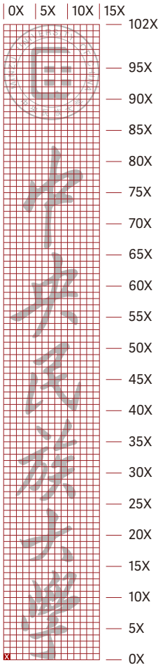
图形标志与竖式中文标志上下组合网格制图
